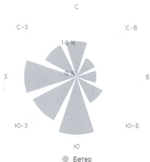
Рисунок 6. Роза ветров МО Алапаевское
