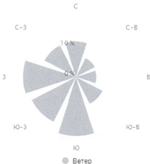
Рисунок 2. Роза ветров МО Алапаевское
