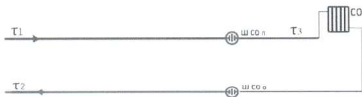
Рисунок 3. Схема присоединения теплопотребляющих установок
