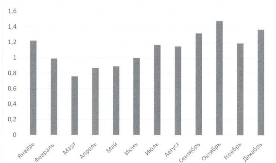
Рисунок 1. Средняя скорость ветра на территории МО Алапаевское в течение года
