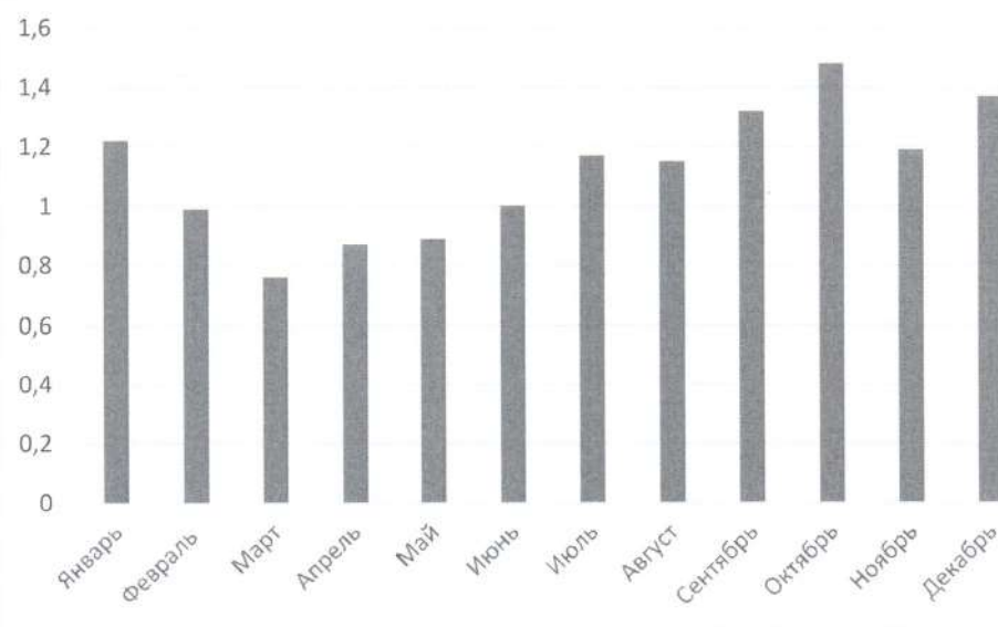
Рисунок 5. Средняя скорость ветра на территории МО Алапаевское в течение года
